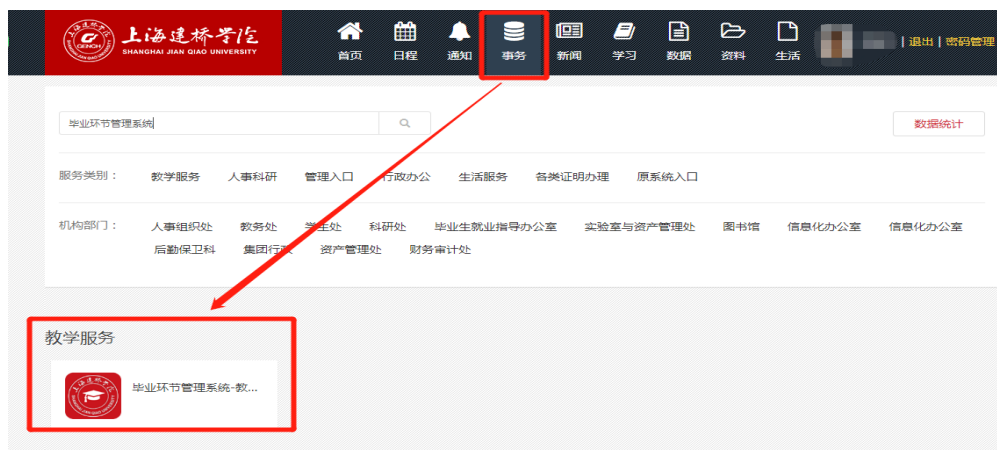
图 4.1 登录界面
