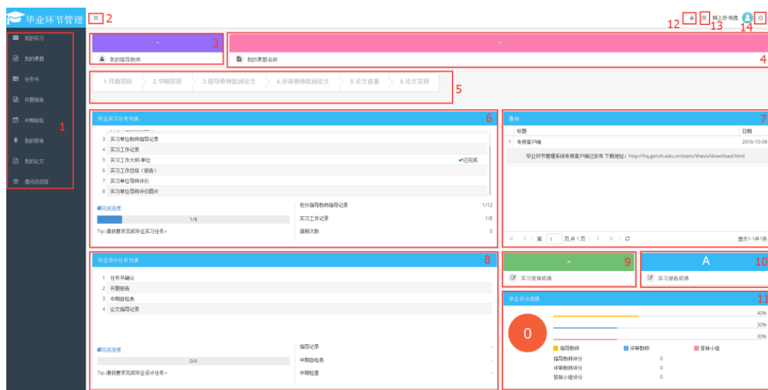
图 4.2 系统首页
